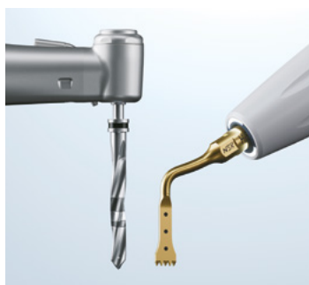
Kobling mellom Surgic Pro2 og VarioSurg 4
